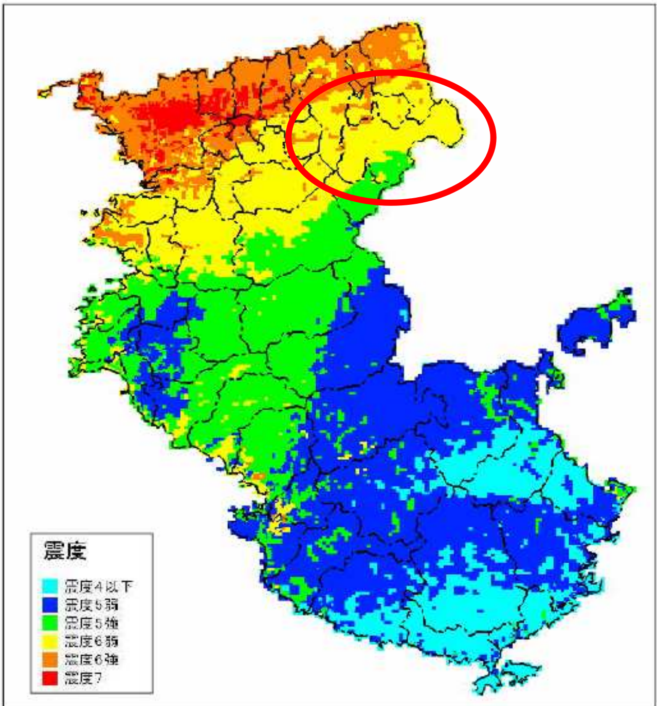
図1 震度分布予測結果（中央構造線による地震）
